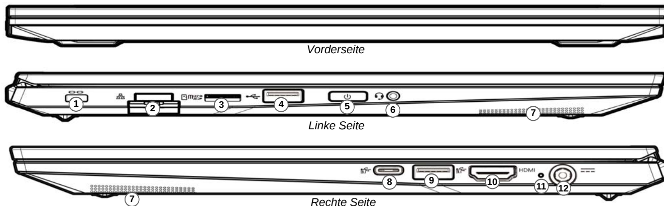
Abb. 9 - Ansicht von vorne, links und rechts (Modell A)
