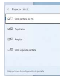
Figura 15 Proyectar
