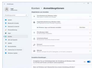
Abb. 20 - Konten - Anmeldeoptionen
