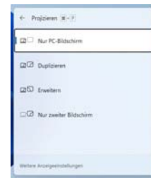
Abb. 15 Projizieren
