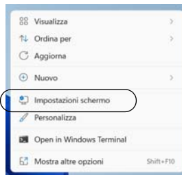
Figura 14 - Impostazioni schermo
