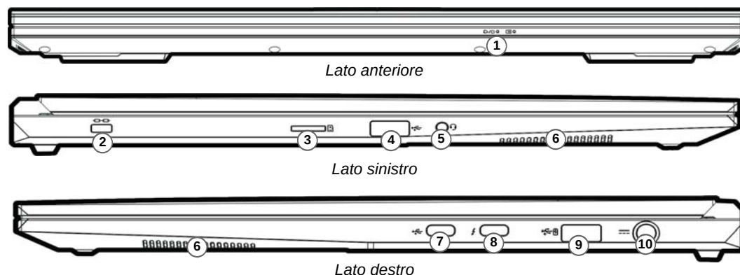
Figura 8 - Vista anteriore, sinistra e destra (Modello B)
