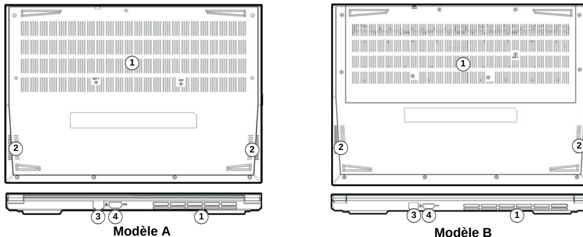
Figure 9 Vues de dessous et arrière
