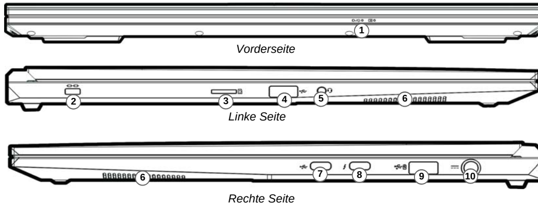
Abb. 8 - Ansicht von vorne, links und rechts (Modell B)
